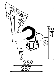
Montaža na špirovce Under-roof installation
