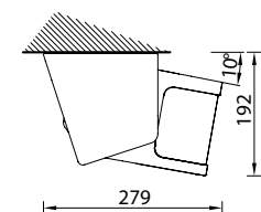
Stropna montaža 80° Ceiling installation 80°
