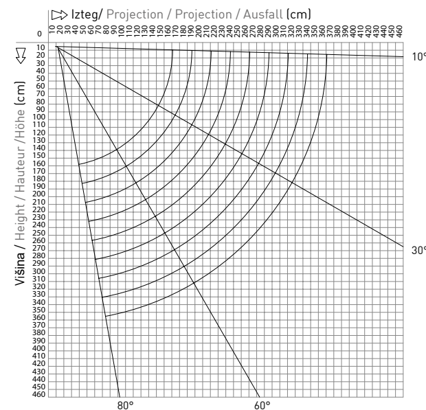
Stropna montaža 80° Ceiling installation 80°
